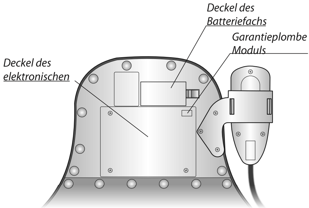
Abbildung 2. Modul für Elektrostimulation (Untenansicht des den elektronischen Baustein enthaltenen Teils)
