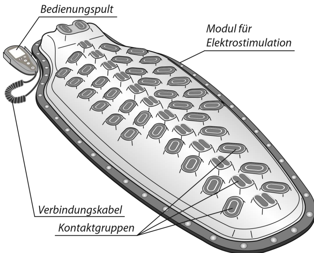
Abbildung 1. Zusammengebautes Gerät. Oberansicht
